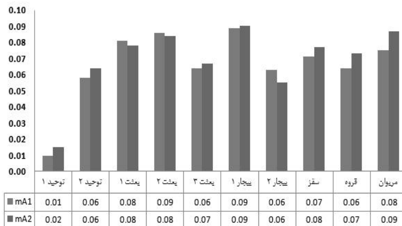
نمودار ۶: درصد خطا در خطی بودن خروجی تیوب نسبت به mA به تفکیک مراکز
