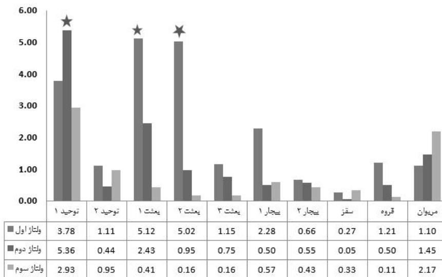
نمودار ۱: درصد خطا در صحت ولتاژ به تفکیک مراکز
