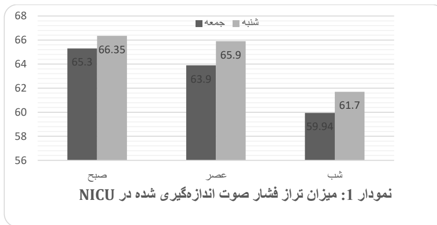
نمودار ۱. میزان تراز فشار صوت اندازه‌گیری شده در NICU
