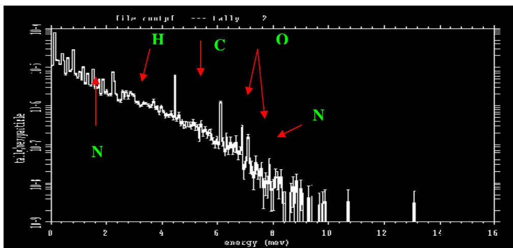
شکل (۳): طیف انرژی گامای حاصل از فعال سازی با منبع طیف شبیه ماکسول (رآکتور)
